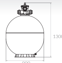
VC-250 TOP
